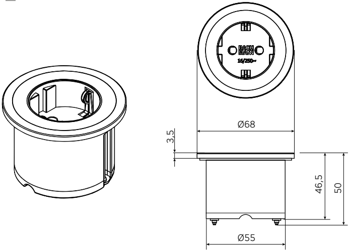
Диаметр монтажного отверстия 56мм.
