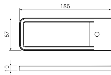
Lineo TDM Мастер-светильник
