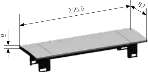
Очень простой скрытый монтаж
