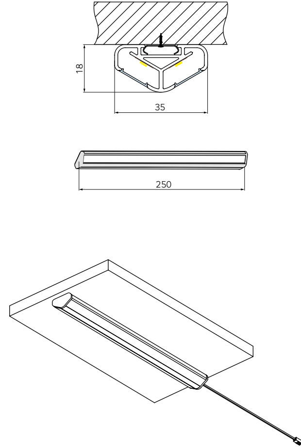
Светильник Tetra оригинальной конструкции — с парой линейных Led-источников — обеспечивает яркую подсветку с широкой областью покрытия. При установке светильника торцом вплотную к стене кабель проводится за стенкой шкафа.
